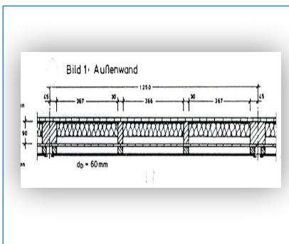
Abb. 34: 1970 Holzbauweise mit 3 cm Luftschicht, die Dämmdicken wachsen
