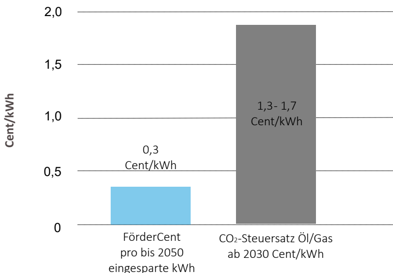
Ab. 112: FörderCent pro eingesparte kWh bis 2050 und CO 2 -Steuerbelastung pro verbrauchter kWh Öl und Erdgas - Einblasdämmung in Dachböden
