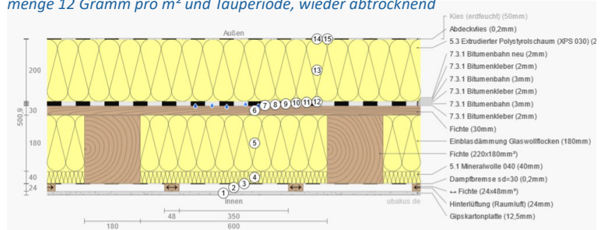
Abb. 126: Kombidach mit Umkehrdach und Volldämmung, U 0,1 W/(m 2 K), Tauwassermenge 12 Gramm pro m 2 und Tauperiode, wieder abtrocknend
