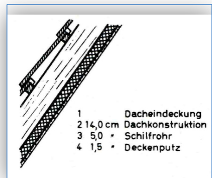
Abb. 72: 1963 Schilfrohr als Dämmung und Putzträger, große Luftschicht
