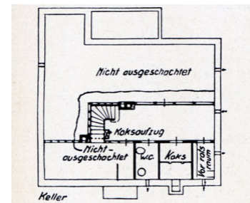
Abb. 61: Kellergrundriss von 1934
