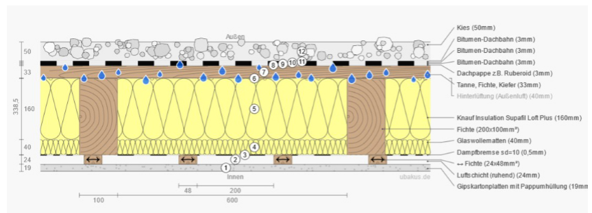
Abb. 125: Flachdach-Volldämmung im Belüftungsraum, U = 0,21 W/(m 2 K) und Tauwasserausfall 120 Gramm/m 2 und Tauperiode nach DIN 4108, wieder abtrocknend
