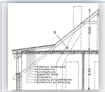
Abb. 85: Ab 1800 Dünne Sandschüttung
