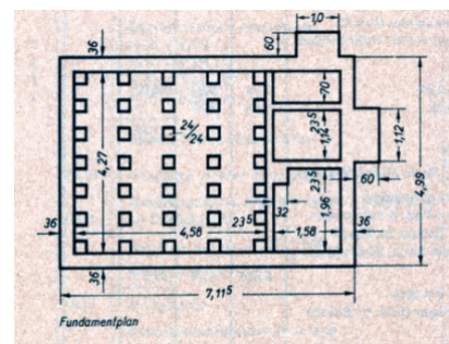
Abb. 62: Fundamentplan für einen Kriechkeller 1968
