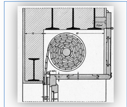
Abb. 138: Rollladenkasten aus der Gründerzeit noch im Betrieb U = 3,0 \text{ W}/(\text{m}^2\text{K})
