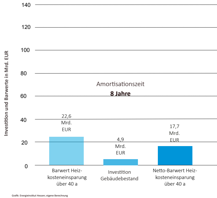
Abb. 89: Investitionskosten und Barwert der Heizkosteneinsparung in Mrd. EUR durch Einblasdämmung auf Kehlbalkenlagen im Wohngebäudebestand
