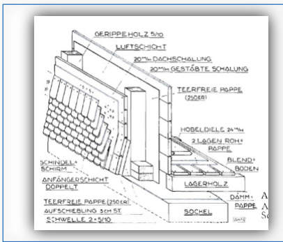
Abb. 31: 1920 ff Holzbauweisen mit 10 cm Luftschicht oder Torffüllungen usw.
