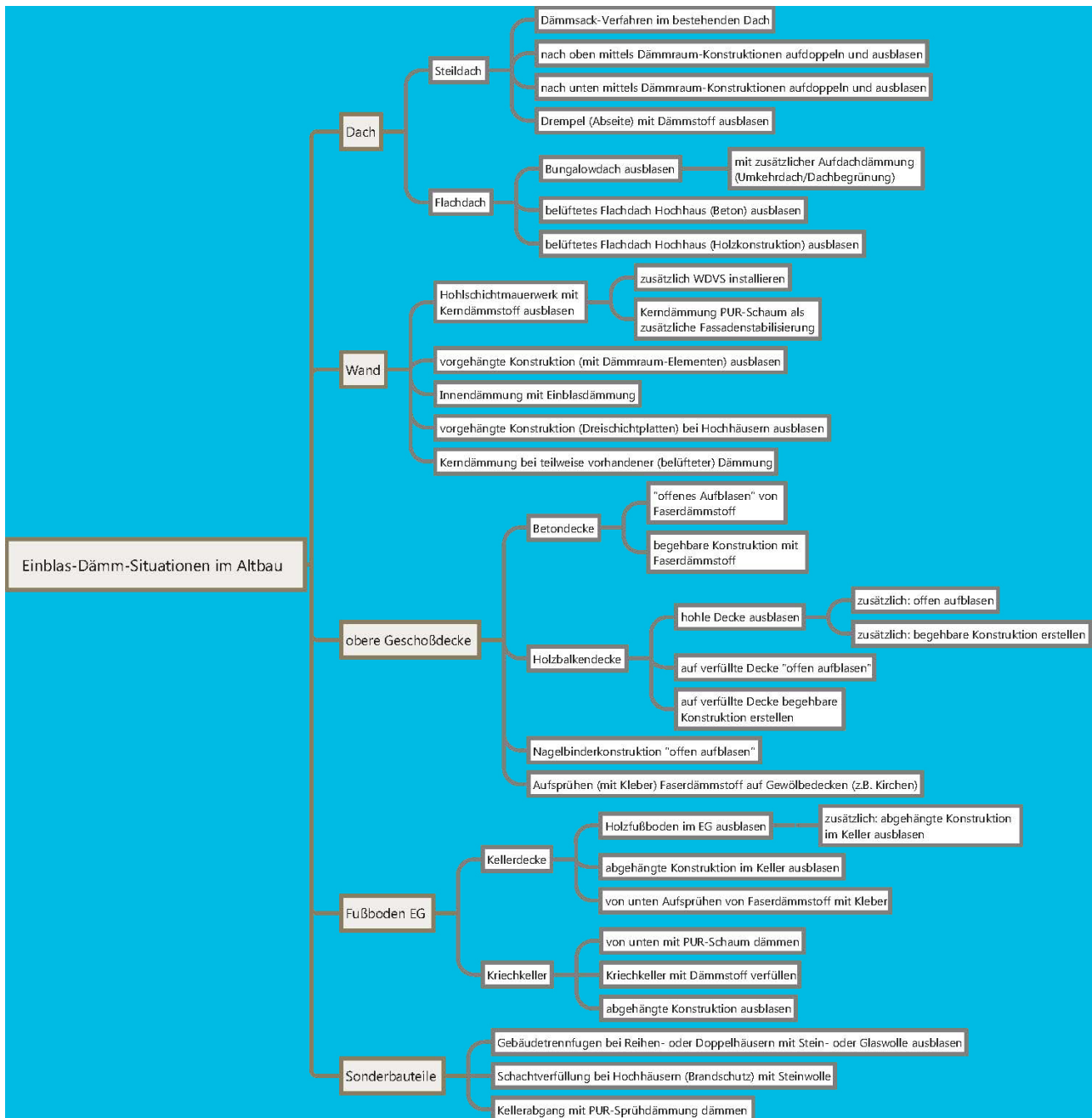
Abbildung 8: 31 Anwendungsfelder der Einblasdämmung
