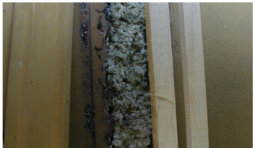
Abb. 149: Gedämmte Trennwandfuge
