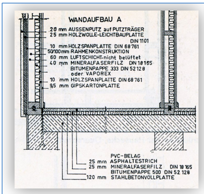
Abb. 33: 1960 Holzständer- und Rahmenbau mit wenig Dämmung und hier z.B. 6 cm Hohlraum
