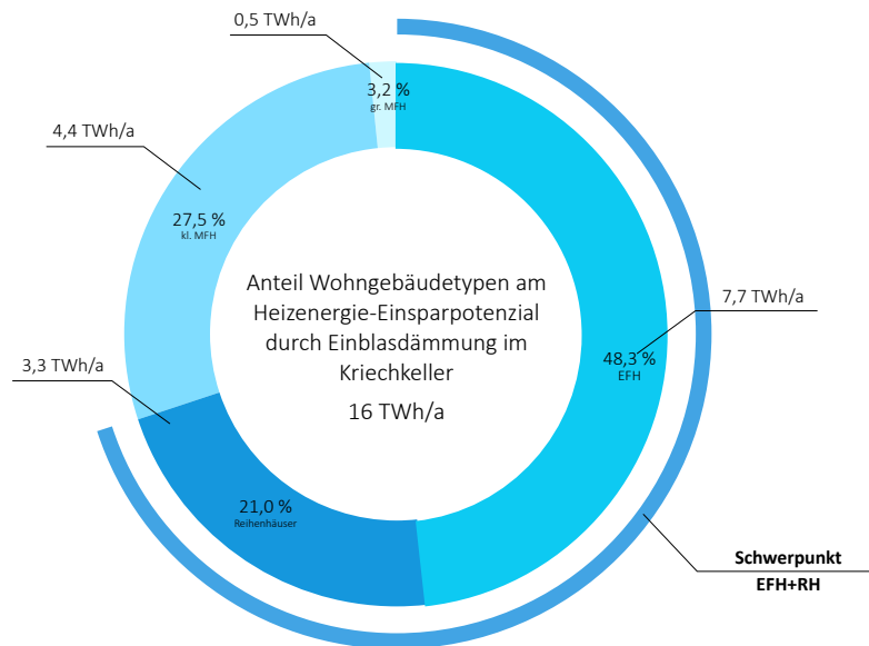
Abb. 63: Heizenergie-Einsparpotenzial durch Einblasdämmung bei Kriechkellern im Wohngebäudebestand in TWh/a und Prozent
