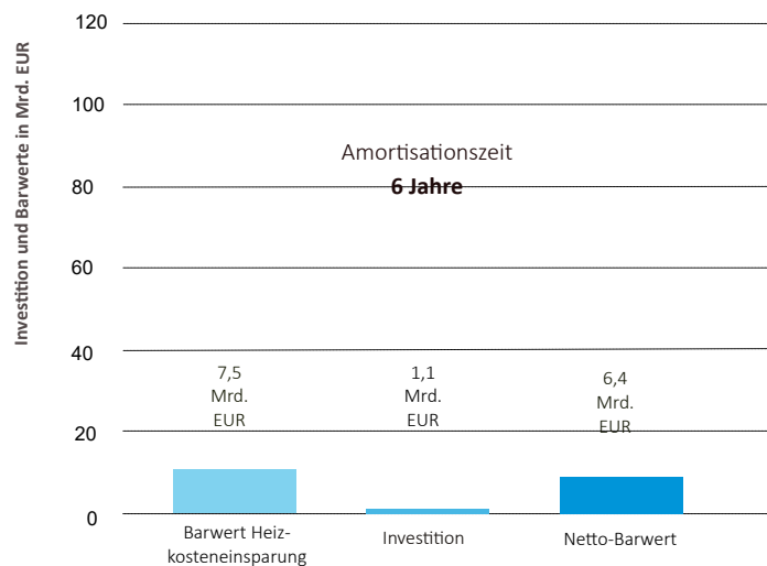
Abb. 121: Investitionskosten und Barwert der Heizkosteneinsparung bei Einblasdämmung in belüftete Flachdächer
