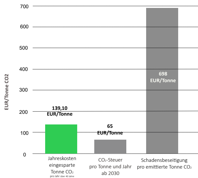
Abb. 64: Einblasdämmung bei Kriechkellern - Kosten der eingesparten Tonne CO 2 im Vergleich im Wohngebäudebestand
