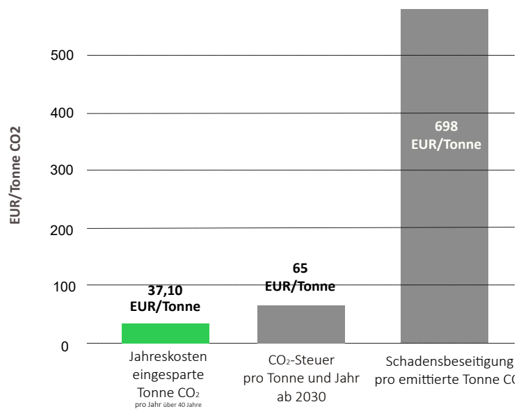
Abb. 25: Kosten der eingesparten Tonne CO 2 im Vergleich - Innendämmung von Fachwerkwänden.
