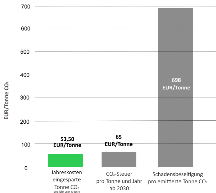
Abb. 134: Kosten der durch Einblasdämmung in belüftete Betonflachdachkonstruktionen eingesparten Tonne CO 2 im Vergleich
