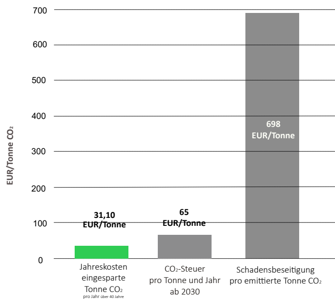
Abb. 120: Kosten der eingesparten Tonne CO 2 durch Einblasdämmung im Belüftungsraum von Flachdächern im Vergleich
