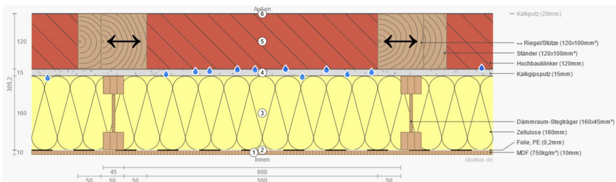
Abb. 23: Fachwerkkinnendämmung mit Stegträger, feuchtetechnisch OK mit diffusionshemmender fugendichter Innenbekleidung
