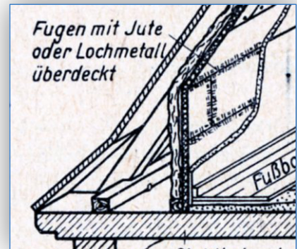
Abb. 92: 1950 ff. Fehlende Dämmung auf der Decke der Abseite
