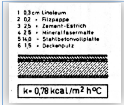
Abb. 103: BMBau Schriftenreihe 1978 Dachböden aus Modellbauvorhaben 0,91 \text{ W}/(\text{m}^2\text{K})
