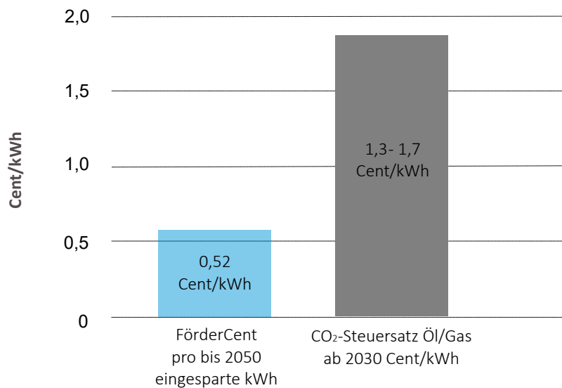
Abb. 82: FörderCent pro bis 2050 eingesparte kWh Heizenergie im Vergleich mit CO 2 -Steuer - Dachschrägendämmung mit dem Thermo-Bag
