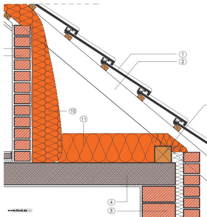
Abb. 97: Abseitendämmung kombiniert mit Thermo-Bag
