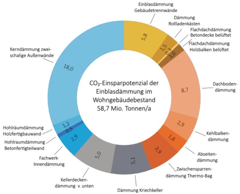
Abb. 1: CO 2 -Einsparpotenzial durch Einblasdämmung nach Bauteilen im Wohngebäudebestand
