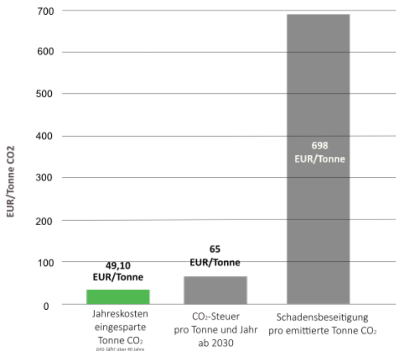
Abb 37: Kosten der eingesparten Tonne CO 2 im Vergleich - Einblasdämmung in Fertighausaußenwände
