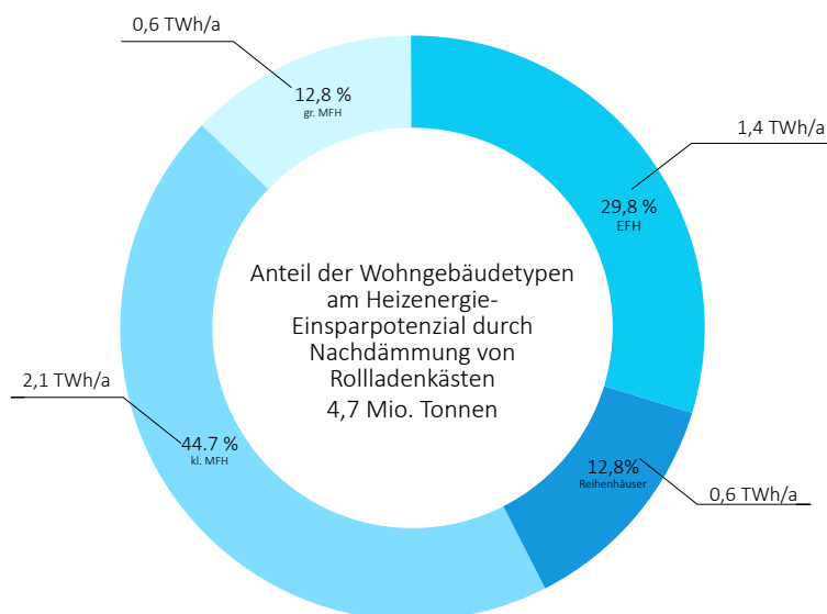
Abb. 141: Heizenergie-Einsparpotenzial durch Nachdämmung von Rollladenkästen im Gebäudebestand in TWh/a und Prozent
