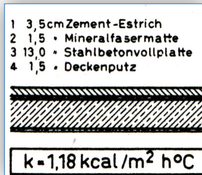
Abb. 106: BMBau Schriftenreihe 1978 Dachböden aus Modellbauvorhaben 1968 1,37 \text{ W}/(\text{m}^2\text{K})
