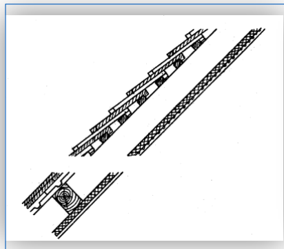
Abb. 70: 1920 ff. Torfplatten unter den Sparren
