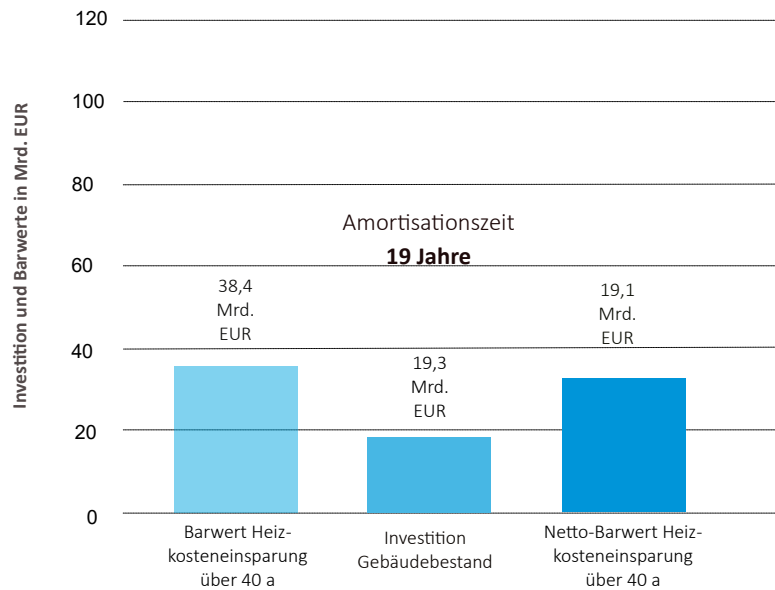
Abb. 57: Kellerdecken-Einblasdämmung - Investitionskosten und Barwert der Heizkosteneinsparung in Mrd. EUR
