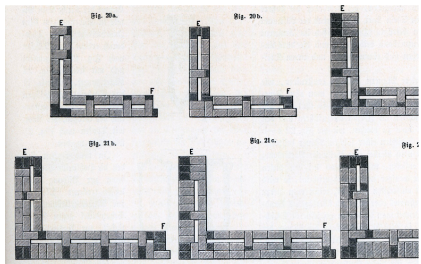
Abb. 12: Die häufigsten „Hohlmauer“-Arten 1881
