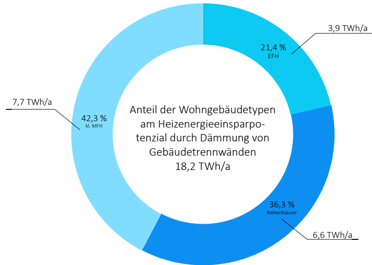
Abb. 150: Heizenergie-Einsparpotenzial durch Einblasdämmung in Gebäudetrennwandfugen in TWh/a und Prozent nach Gebäudetypen
