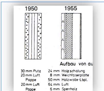
Abb. 32: 1950 Erste Erfahrungen, 2*2,0 und 6 cm Luftschichten waren dabei
