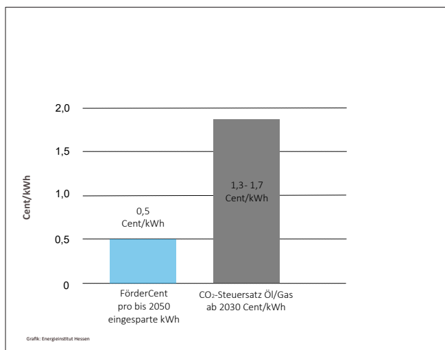
Abb. 129: FörderCent pro bis 2050 eingesparte kWh Heizenergie im Vergleich - Flachdachvollämmung
