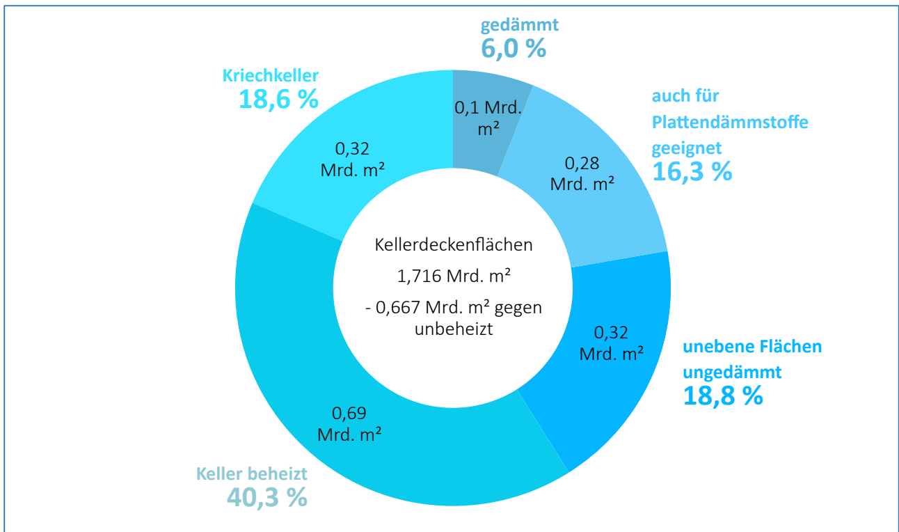
Abb. 52: Verteilung der Kellerdeckenflächen nach Nutzung und Dämmstatus im Wohngebäudebestand
