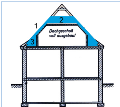
Abb. 68: 3 Einsatzbereiche der Einblasdämmung im Steildach
