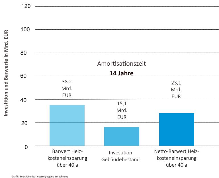
Abb. 65: Investition und Barwert der Heizkosteneinsparung in Mrd. EUR - Dämmung von Kriechkellern
