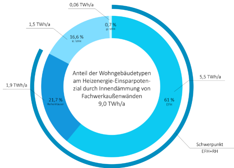
Abb. 24: Heizenergie-Einsparpotenzial der Einblasdämmung bei Innendämmung von Fachwerkaußenwänden nach Gebäudetypen in TWh/a
