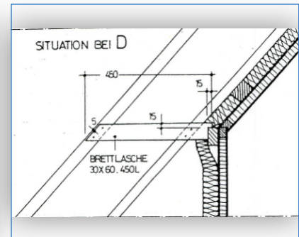
Abb. 74: 1977 Fertighausdach mit Stegträgern, dem Passivhausstandard steht nichts im Wege
