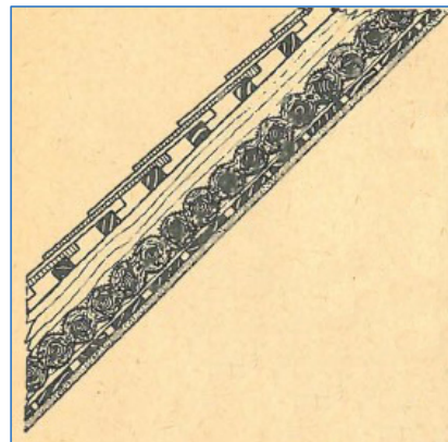
Abb. 69: 1890 ff. Lehmstakung lässt Luft für Einblasdämmung
