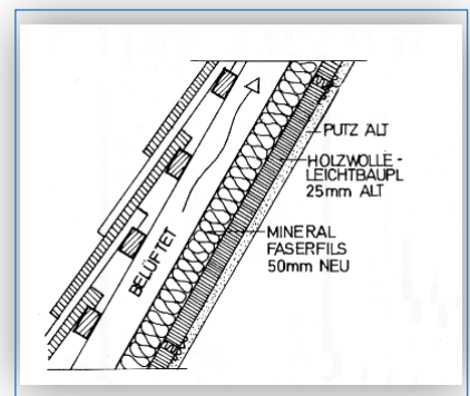
Abb. 73: 1975 zaghaft gedämmt, 2022 noch Luft für die Einblasdämmung
