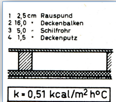
Abb. 105: BMBau Schriftenreihe 1978 Dachböden aus Modellbauvorhaben 1968 0,59 \text{ W}/(\text{m}^2\text{K})
