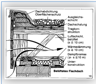
Abb. 114: Flachdach 1960 hoher Stegräger mit wenig Dämmung
