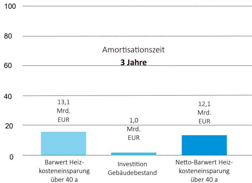
Abb. 100: Investitions- und Barwertsummen in Mrd. EUR bei der Einblasdämmung in Abseitenräume im Wohngebäudebestand
