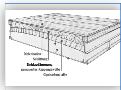
Abb. 51: 1890 ff. Kappendecke, bereits mit Einblasdämmung von unten gedämmt
