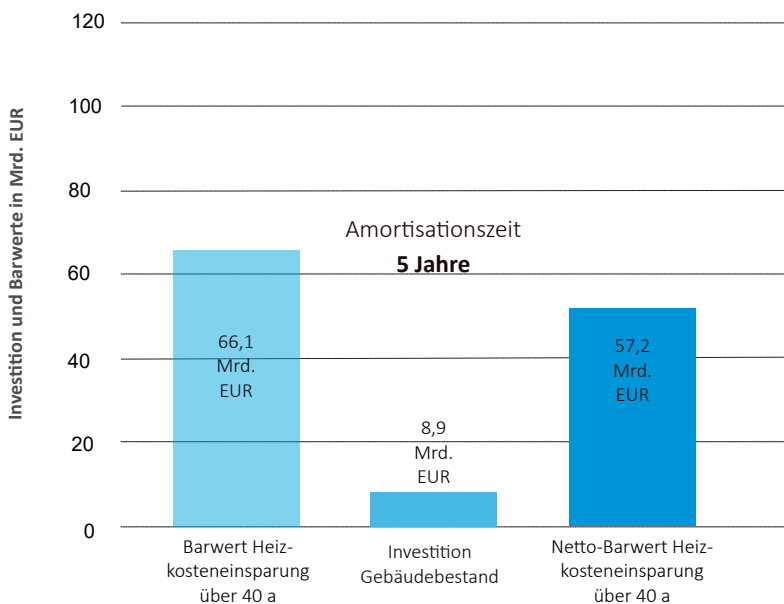
Ab. 111: Investitions- und Barwertsumme in Mrd. EUR bei der Einblasdämmung Dachböden im Wohngebäudebestand
