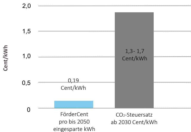
Abb. 18: FörderCent pro bis 2050 eingesparte kWh Heizenergie im Vergleich - Kerndämmung im Wohngebäudebestand
