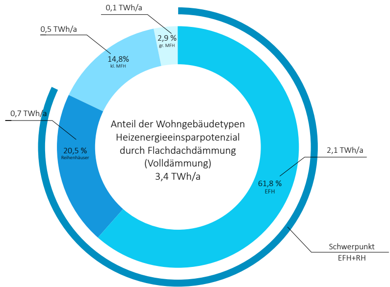
Abb. 124: Heizenergie- Einsparpotenzial durch Einblasdämmung in bel. Flachdächer (Volldämmung) im Gebäudebestand in TWh/a und Prozent
