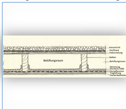
Abb. 115: Balkenflachdach 1960 mit 3-6 cm Dämmung U = 0,61-0,97 \text{ W}/(\text{m}^2\text{K})
