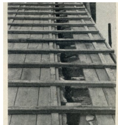
Abb.13: Ortgang offen wg. Hohlchicht
