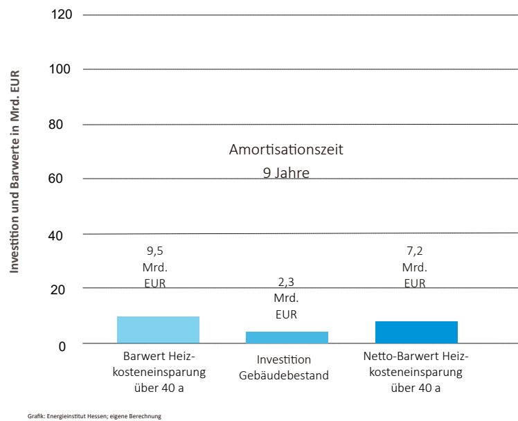
Abb. 38: Investitionskosten und Barwert der Heizkosteneinsparung über 40 Jahre - Einblasdämmung in Fertighausaußenwände
