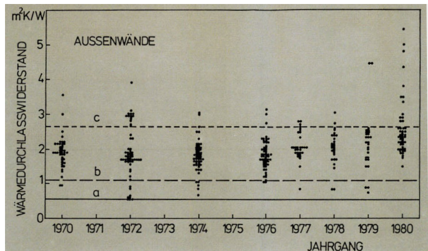
Abb. 30: IBP-Untersuchung Wärmeschutz von Fertighaus-Außenwänden 1970 bis 1980 als Wärmedurchlasswiderstand
