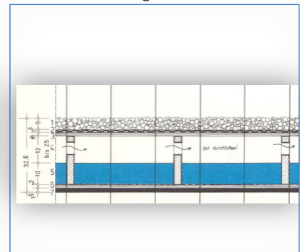
Abb. 116: 1978 besser als gefordert mit 10 cm Dämmung, 12 cm Belüftung U = 0,35 \text{ W}/(\text{m}^2\text{K})
