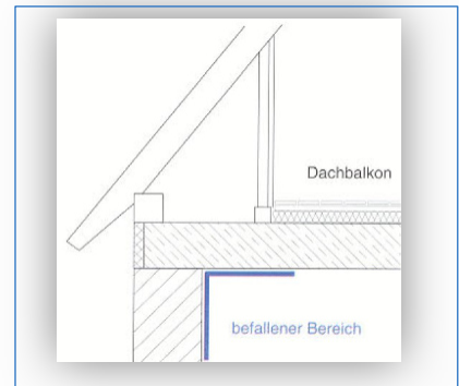
Abb. 93: 1990 Abseitenraum Schimmel unter ungedämmter Stahlbetondecke
