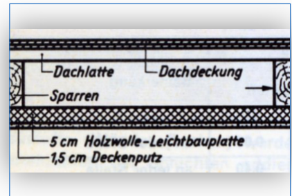
Abb. 71: 1920 ff. Klassiker Holzwolleleichtbauplatte mit 10 - 14 cm Luftschicht
