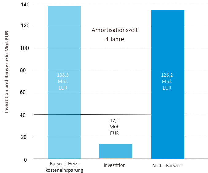
Abb. 17: Investitionen und Barwert in Mrd. EUR - Kerndämmung im Wohngebäudebestand
